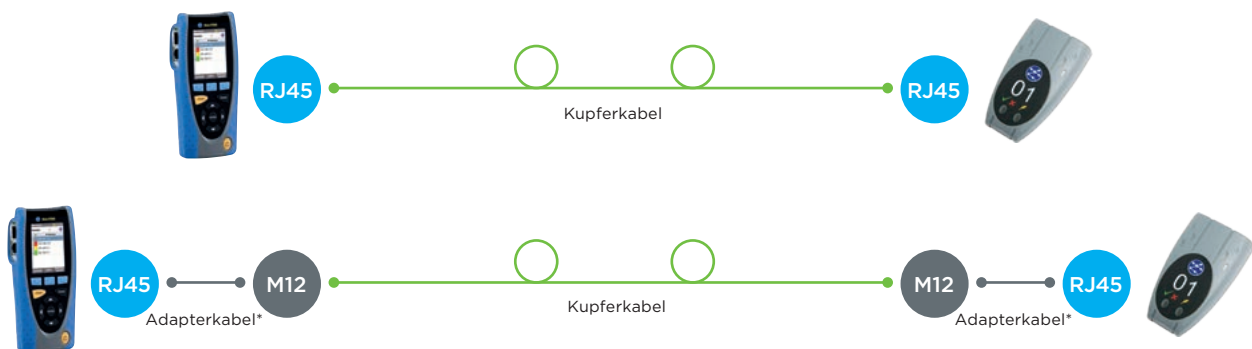
2 x Kabel mit M12-Stecker (D-kodiert) im Lieferumfang enthalten. M12-Stecker (X-kodiert) als Zubehör erhältlich.
